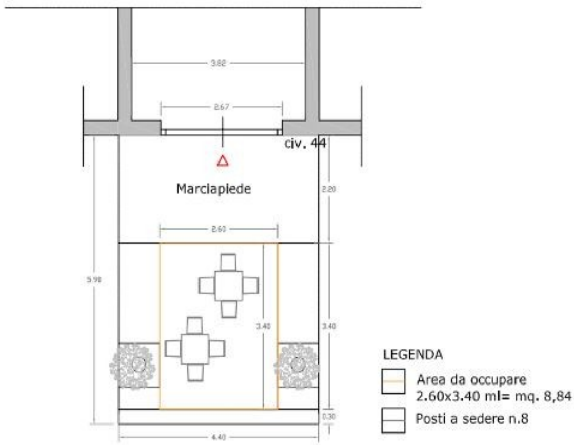
Planimetria dello stato di Progetto
