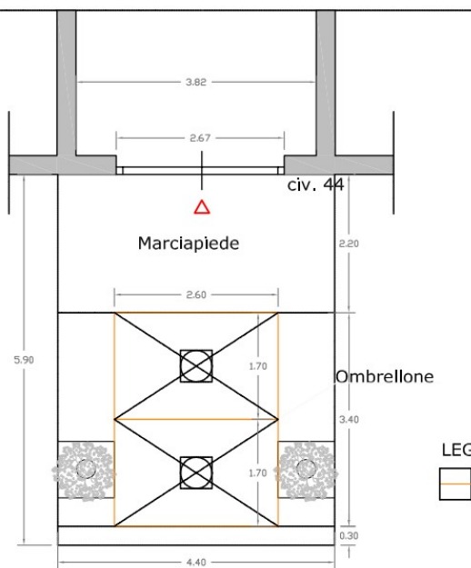
Planimetria dello stato di Progetto
