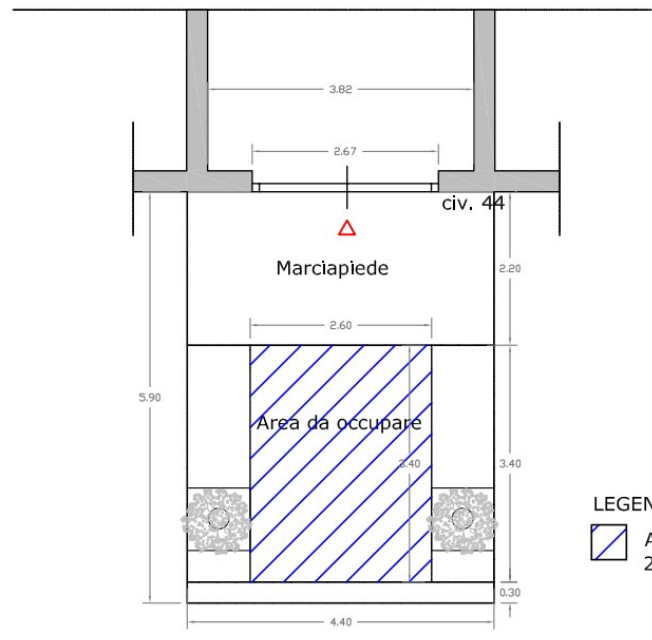
Planimetria dello stato di Progetto
